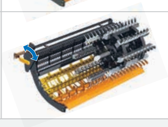
Batteur universel et contre-batteur à riz à sections
