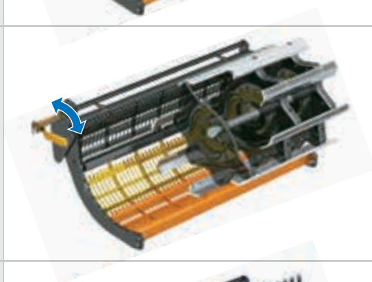
Batteur standard et contre-batteur à maïs à sections
